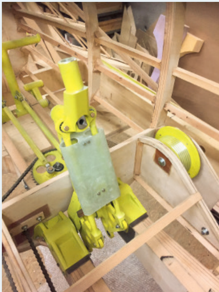
Ausschnitt aus dem Rumpfhohbau mit eingebauter Steuerknüppelkinematik. | Détail du gros-œuvre du fuselage avec cinématique intégrée de manche à balai.
